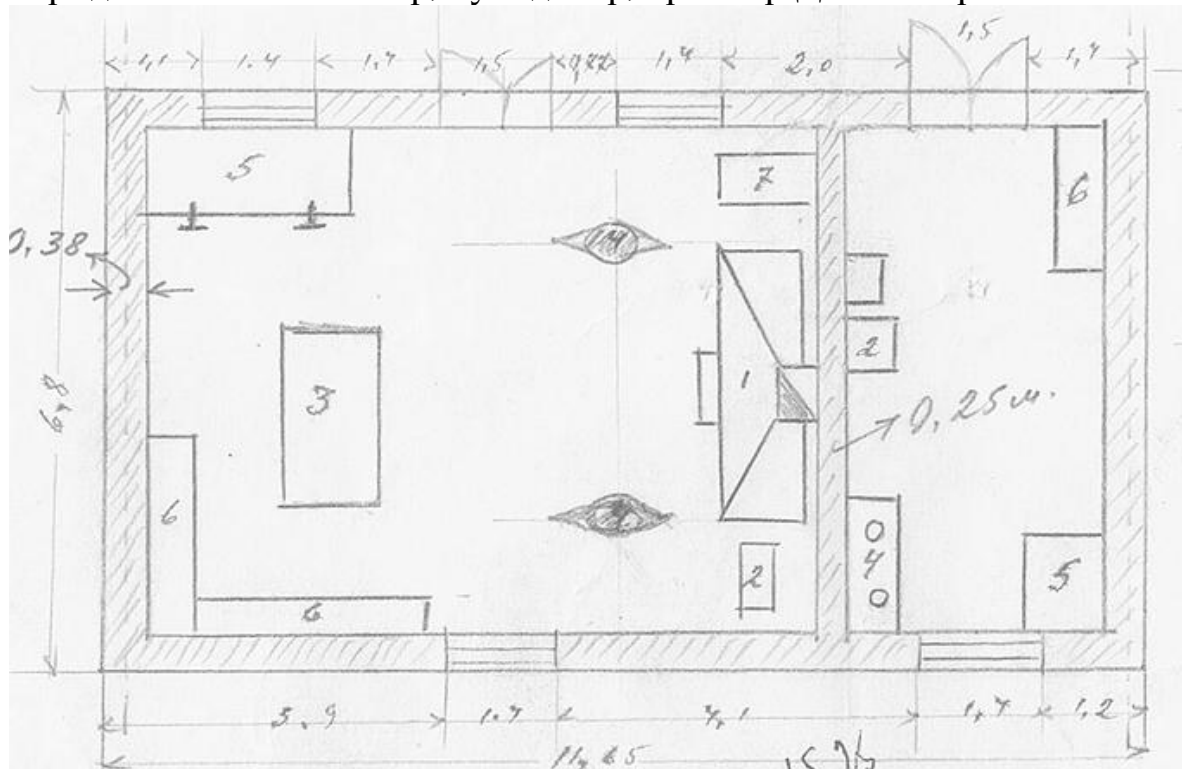
План стен и размещения оборудования простиряемого помещения под сварочный и кузнечный цеха. Приложение к смете 1958г.
