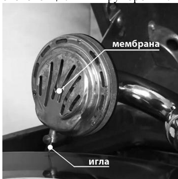
План передачи звука от иглы к резонатору.
