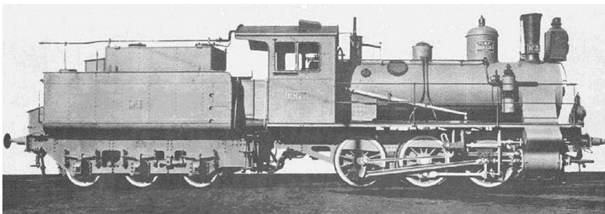
Паровоз серии Т (тип 132 Коломенского завода)
